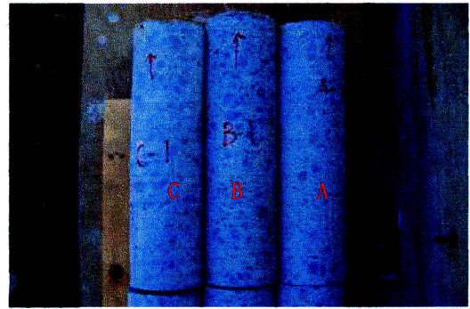
写真-2 骨材の分離状況
