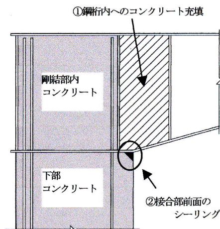
図-3 応力集中対策
