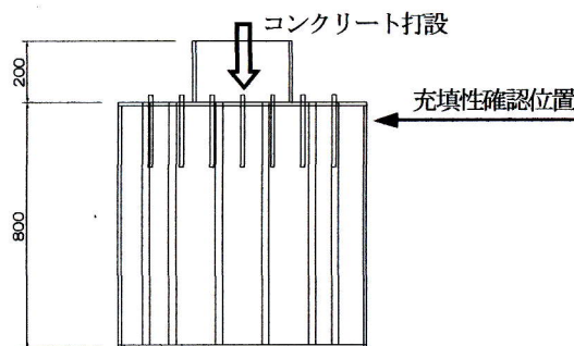
図-7 コンクリートの充填性確認のための試験体
