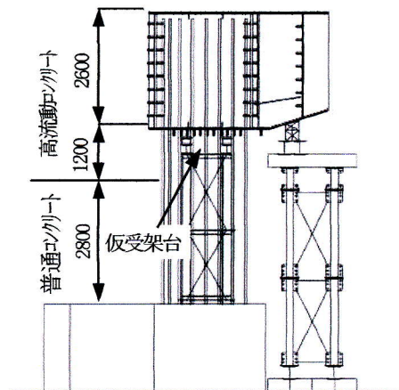
図-9 剛結部の架設
