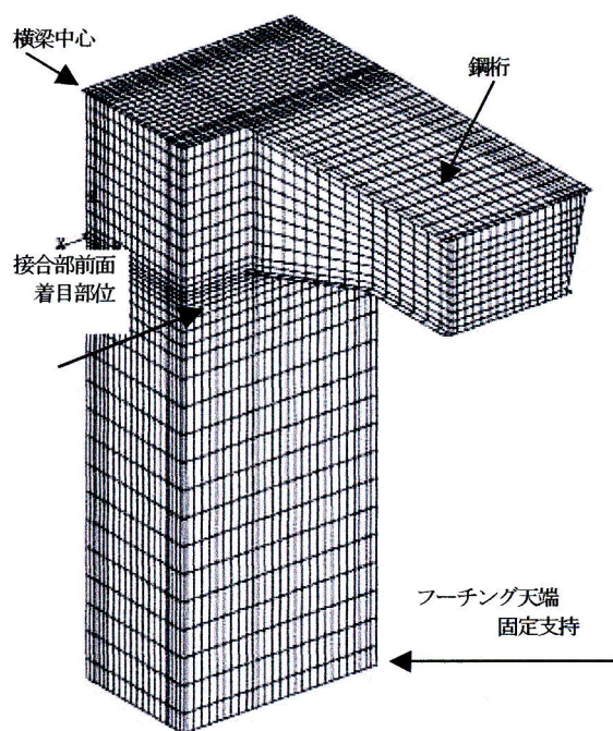
図-4 解析モデル
